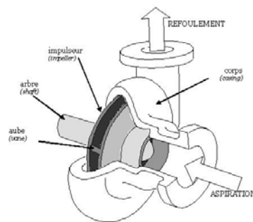
Pompe centrifuge
