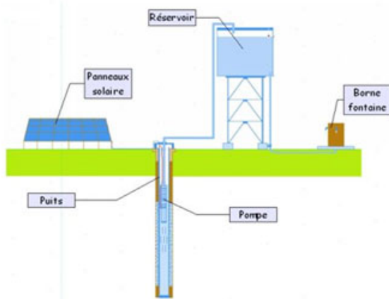
Système de pompage
